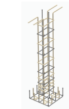
GFRP Column
